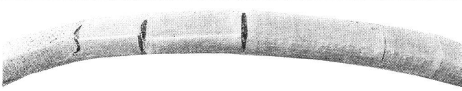
Fig. 3 Durch Strahlung beschädigtes PE-Kabelstück Dosis ca. 3...5 MGy
