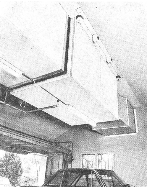
Luftkühler zu Aerocal-Wärmepumpe, an Garagedecke montiert
