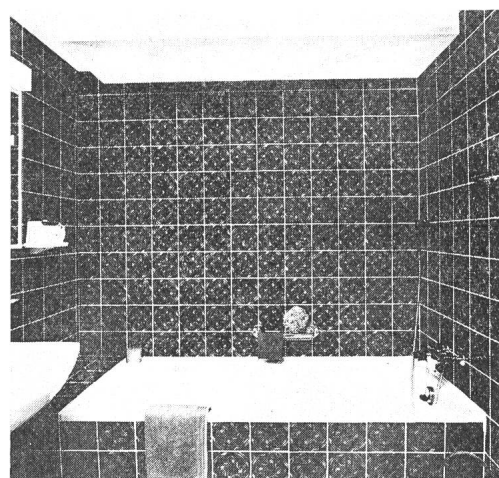
Deckenboiler DW 160, über einer Badewanne eingebaut
