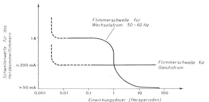
Fig. 6 Prinzipielle Verlauf der Schwellenwerte für das Auslösen von Herzkammerflimmern bei Wechselstrom 50...60 Hz und Gleichstrom, bei Längsdurchströmung
