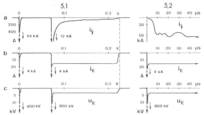
Fig. 5 Beispiel eines negativen Abwärtsblitzes mit zwei Teilblitzen
