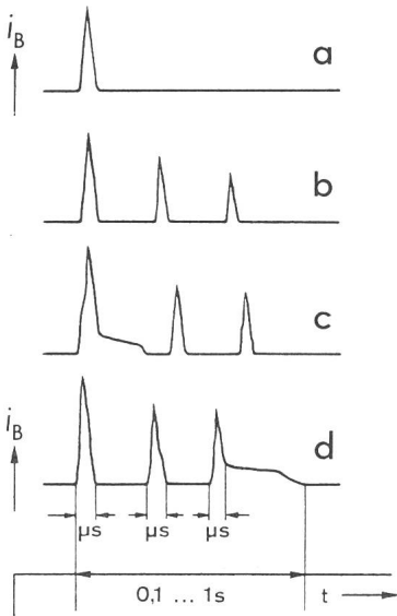
Fig. 4 Prinzipielle Darstellung des Stromverlaufes i_B von Abwärtsblitzen
