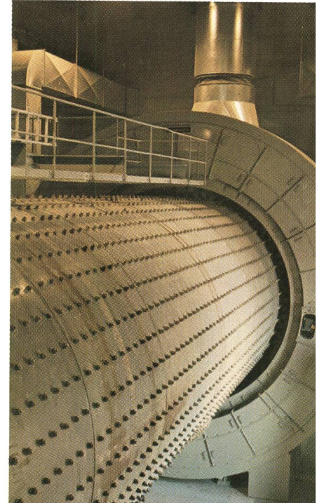
Zementmühlenantrieb Rekingen
