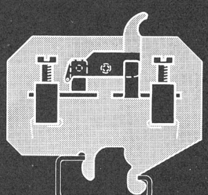
Trennmesserklemme 4 mm 2 , 500 V
