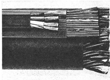
Vieladrige Flachkabel mit Kunststoff- oder BUTANOX-Gummi-Isolation.
