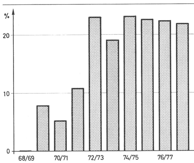
Anteil der Kernenergie an der schweizerischen Gesamtstromerzeugung (ohne Pumpenergie) in den Winterhalbjahren
