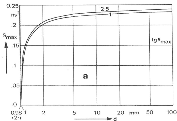
Fig. 10 Maximale Flankensteilheit bezogen auf die Pulsamplitude am Eingang Daten wie in Fig. 8
