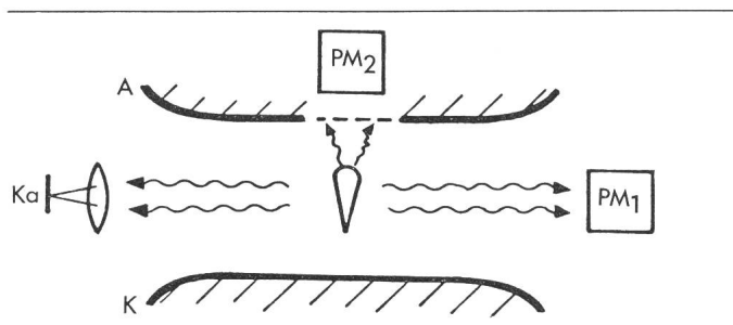
Fig. 3 Zur optischen Erfassung der Lawinenstrahlung im Raum zwischen Kathode (K) und Anode (A) Durch Photomultiplier seitlich (PM 1 ) oder hinter der Anode (PM 2 ) oder mit der Kamera (Ka) bzw. Bildwandler
