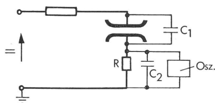
Fig. 2 Schema der elektrischen Aufnahmemethode C_1 Eigenkapazität der Entladestrecke C_2 Eingangskapazität des Verstärkers C \approx C_1 + C_2 wirksame Kapazität
