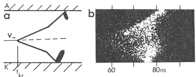
Fig. 18 Integrierende Bildwandlernaufnahme der Kanalaus-bildung
