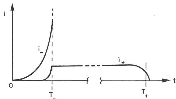
Fig. 1 Elektronen- ( i_- ) und Ionenkomponente ( i_+ ) der Lawine
