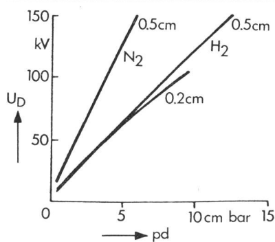
Fig. 23 Paschendarstellung der Durchbruchspannungen in den Gasen Stickstoff und Wasserstoff [26] d = 0,5 \text{ cm} bzw. 0,2 \text{ cm}
