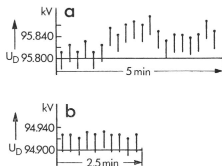
Fig. 22 Streuung der Durchschlagspannung bei aufeinanderfolgenden Zündungen [26] N_2 , 6,7 bar, d = 0,5 cm a unbestrahlt b UV-bestrahlt
