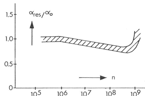
Fig. 11 Ionisierungszahl \alpha_{\text{res}} , bezogen auf \alpha_0 des raumladungsfreien Feldes, in Abhängigkeit von der Lawinengrösse [9] \text{N}_2 , 530 mbar, d = 3 \text{ cm} , 10^3 Startelektronen
