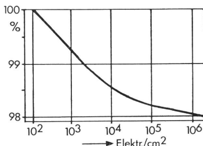
Fig. 21 Absenkung der statischen Durchschlagspannung in Luft mit der Menge der zur gleichen Zeit in der Kathode ausgelösten Anfangselektronen [25] d = 15 cm
