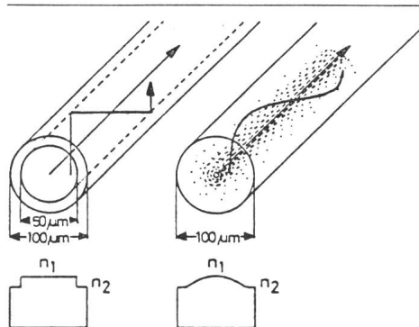
Fig. 4 Fortpflanzung von Licht in einer Stepindexfaser (links) und einer Faser mit gradiertem Brechungsindexprofil
