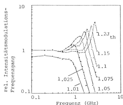
Fig. 4 Gemessener relativer Intensitätsmodulations-Frequenzgang des CSL für verschiedene Laserströme J
