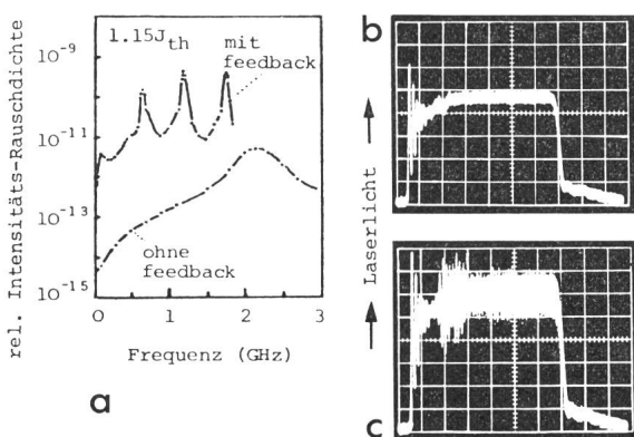
Fig. 10 Einfluss von externem optischem Feedback auf das Rausch- und Einschaltverhalten des Channel-Substrate-Laser
