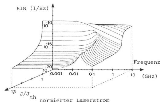
Fig. 6 Theoretischer Verlauf der relativen Intensitäts-Rauschdichte (RIN) für einen Monomode-Diodenlaser
