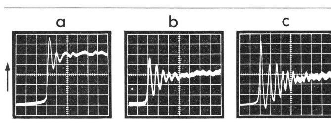
Fig. 5 Einfluss des aktiven Laservolumens auf das Einschwingverhalten des Laserlichts bei identischer normierter Aussteuerung des Lasers mit einem Stromimpuls
