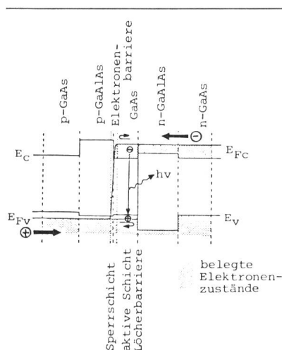
Fig. 2 Schematisches Bandkantenenergiediagramm des Doppelheterostruktur-Diodenlasers bei Vorspannung der Diode in Flussrichtung
