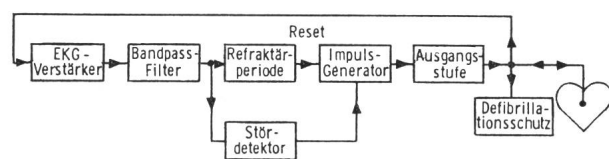
Fig. 5 Blockschaftbild eines Bedarfschrittmachers
