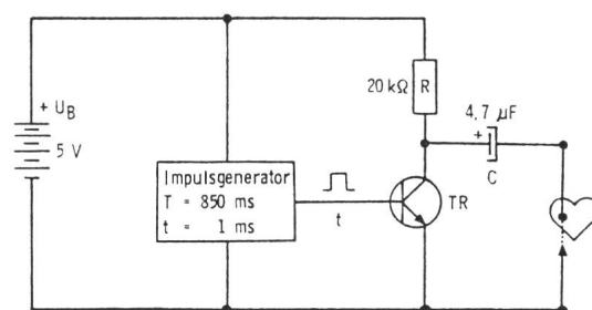
Fig. 4 Funktionsprinzip eines festfrequenten Schrittmachers
