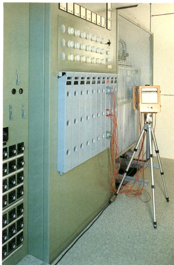
Schalttafel, Messzange mit Punktschreiber
