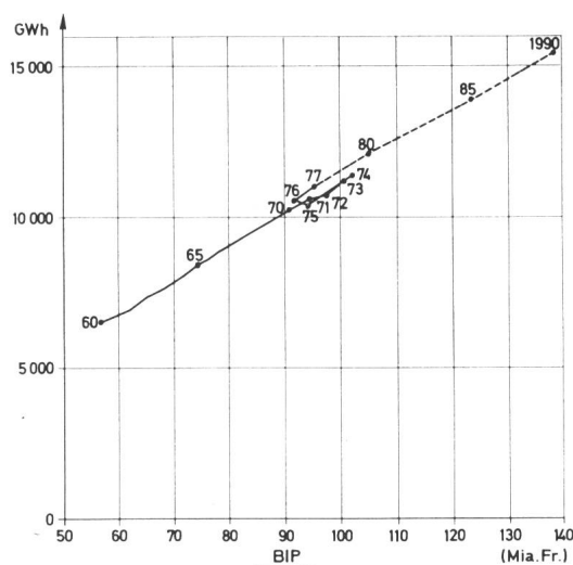
Fig. 9 Unbeeinflusste Bedarfsentwicklung: Korrelation des Stromverbrauchs in der Industrie mit dem Bruttoinlandsprodukt (BIP)
