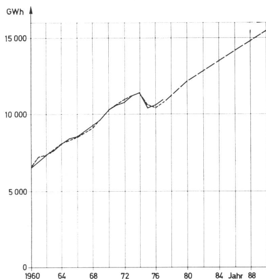
Fig. 8 Unbeeinflusste Bedarfsentwicklung: Stromverbrauch der Industrie (ohne Elektrokessel)
