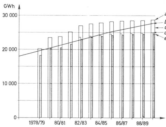
Fig. 3 Strombedarf und Erzeugungsmöglichkeiten im Winterhalbjahr a mittlere Erzeugungsmöglichkeiten b Bedarf c notwendige Reserve d mit 95 % Sicherheit gewährleistete Erzeugungsmöglichkeiten e Erzeugungsmöglichkeiten gemäss dem angepassten GEK-Reservemodell (s. Anhang 18)
