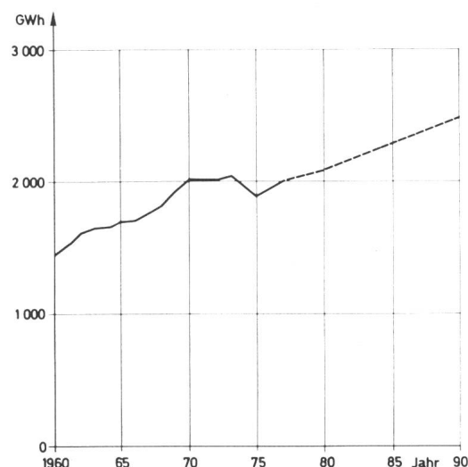
Fig. 10 Unbeeinflusste Bedarfsentwicklung: Stromverbrauch der Bahnen
