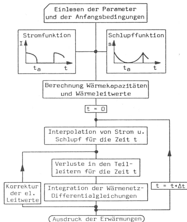
Fig. 4 Flussdiagramm der numerischen Berechnungen
