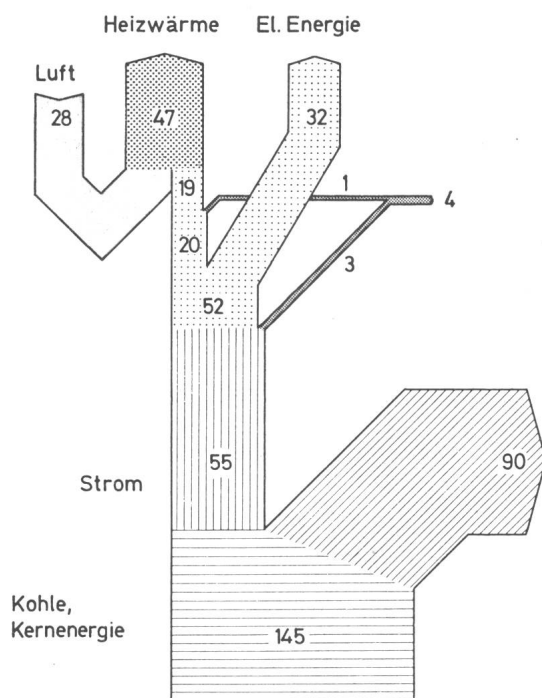
Fig. 2 Wärme- und Stromerzeugung mit Wärmepumpe und Kraftwerk
