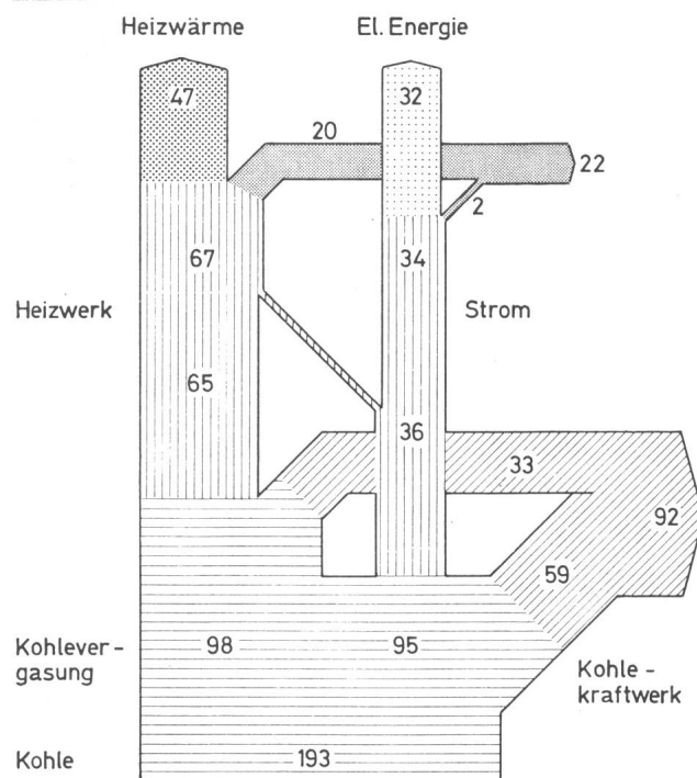
Fig. 3 Wärmeerzeugung über Kohlevergasung und Heizwerk sowie Stromerzeugung im Kohlekraftwerk
