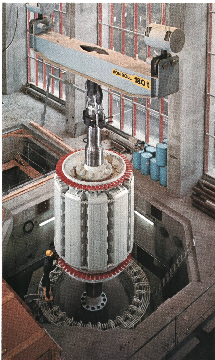
Montage eines der drei Motor-Generatoren des Pump-Speicherwerkes Mapragg der Kraftwerke Sarganserland.
