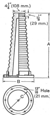
Fig. 11 Innenraumstützisolator aus Porzellan, für höhere Mittelspannung, um 1926 (Ohio Brass)
