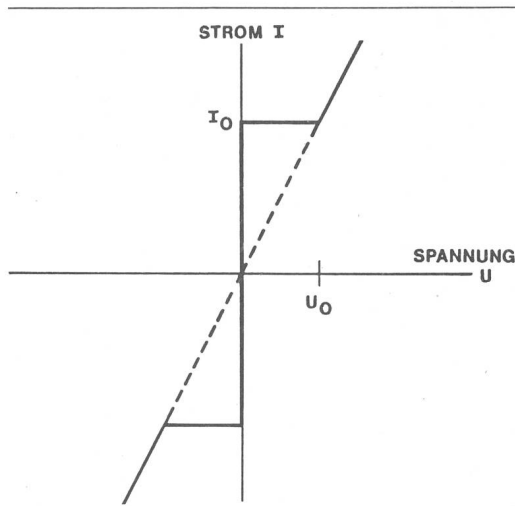
Fig. 2 Strom-Spannungscharakteristik eines Josephsonübergangs
