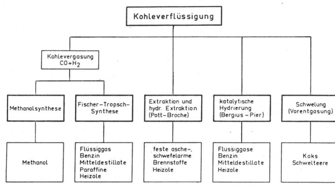
Fig. 14 Kohleverflüssigungsverfahren
