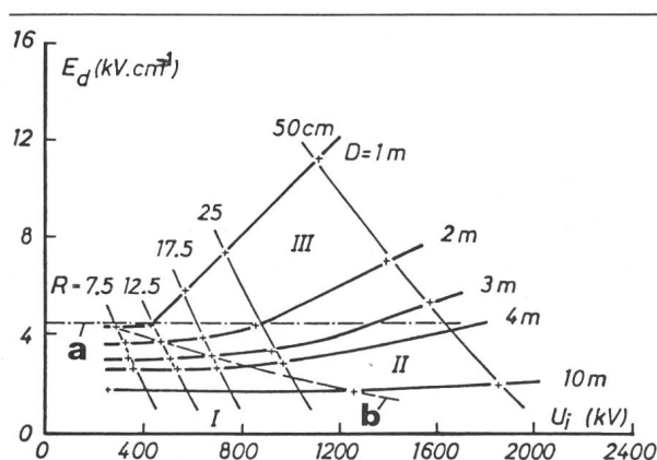
Fig. 7 Mittlerer Durchschlagsgradient E_d einer Kugel-Platte-Funkenstrecke in Abhängigkeit von der Einsatzspannung U_i bei Erscheinen des ersten Koronaeffektes
