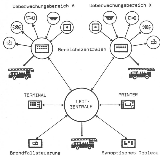
Fig. 2 Hierarchisch gegliedertes Brandschutz-System mit weitgehend autonomen Bereichszentralen und einer Leitzentrale [1]
