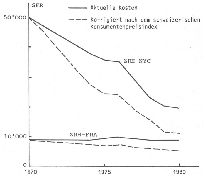
Fig. 3 Monatliche Kostenentwicklung der Mietleitungen Zürich-New York und Zürich-Frankfurt
