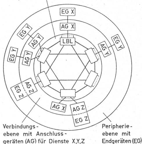
Fig. 5 Systemstruktur SILK
