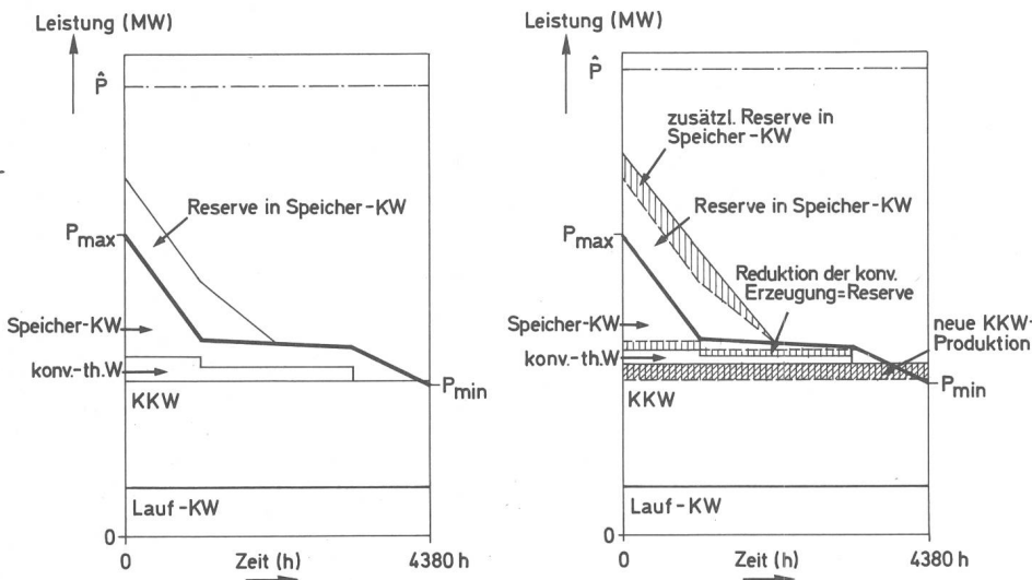
Fig. 7a (links) und 7b (rechts) Bedarfsdeckung und Reserve im Winter Links: Grundannahmen Rechts: bei Zubau eines Kernkraftwerkes \hat{P} : verfügbare Leistung aller Erzeugungsanlagen P_{\max} - P_{\min} : Dauerlinie des Bedarfs
