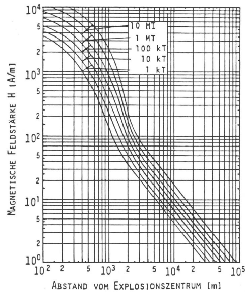
Fig. 6b Maximale magnetische Feldstärken bei Bodenexplosionen
