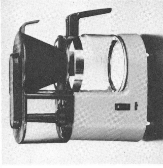
Kaffeeautomat mit Gehäuseteilen aus Novolen (PP), wärmeformbeständig und schlagfest.
