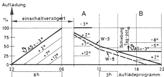
Fig. 9 Aufladesteuergerät für maximal 3 Stunden Tagesnachladung
