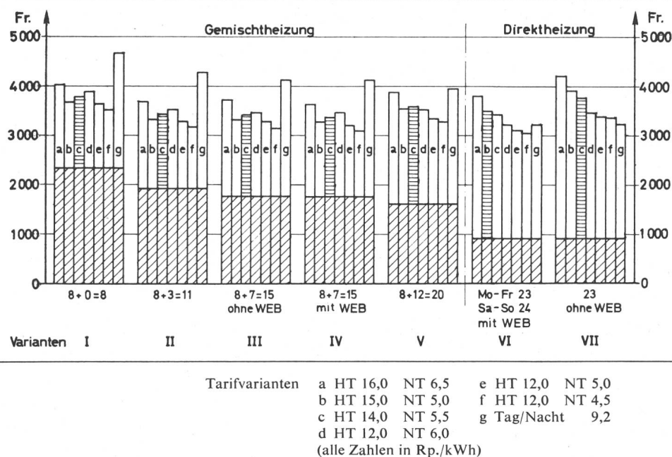
Fig. 8 Einfluss der Tarifgestaltung auf die Jahreskosten für Raumheizanlagen mit unterschiedlichen Nachladezeiten
