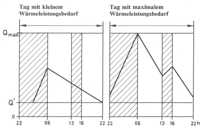
Fig. 5 Aufladecharakteristik bei 3 Stunden Tagesnachladung
