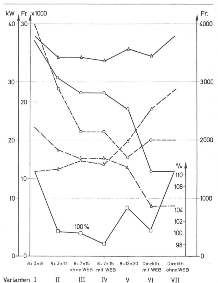
Fig. 7 Jahreskostenvergleich für Raumheizanlagen eines Einfamilienhauses mit unterschiedlichen Nachladezeiten gemäss Tabellen III und IV
