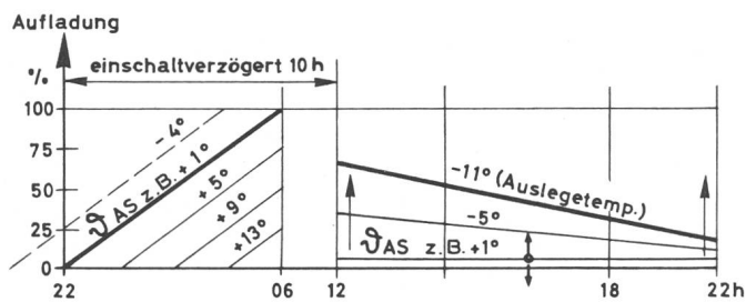
Fig. 11 Aufladesteuergerät für lange Tagesnachladung
