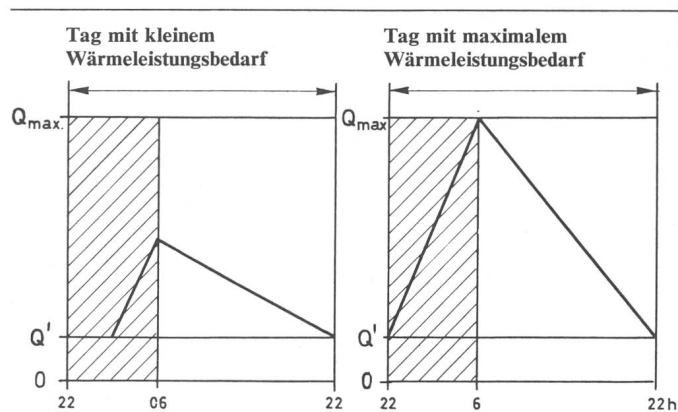
Fig. 4 Aufladecharakteristik ohne Tagesnachladung
