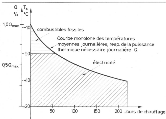
Fig. 2 Fonctionnement bivalent-parallèle
