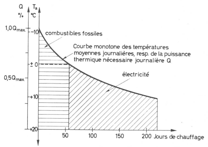
Fig. 1 Fonctionnement bivalent-alternatif
