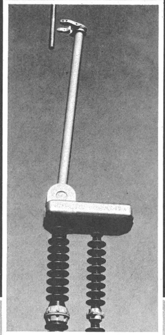
Horizontalgreiftrenner Typ TFN...
