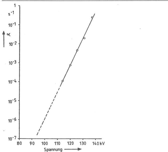
Fig. 4 Durchschlagswahrscheinlichkeitsdichte \alpha in Abhängigkeit von der Spannung, Auswertung von Fig. 3
