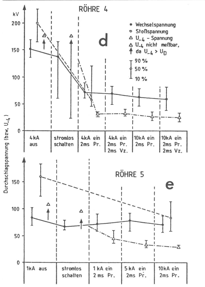
Fig. 2d, 2e Gleich wie Fig. 2a–2c, jedoch Cu/Cr-Kontakte Pr. = Prellen; Vz. = Vorzündlichtbogen
