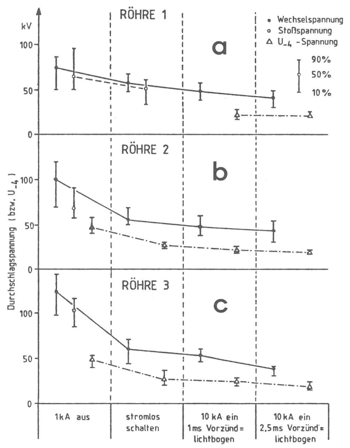
Fig. 2a-2c Durchschlagspannungen und U_{-4} -Spannungen von verschiedenen Vakuumisolerierstrecken nach Ausschaltlichtbögen, stromlosem Schalten und Einschalten verschiedener Ströme, gefolgt von stromlosem Öffnen (Scheitelwerte) Cu/Bi-Kontakte, Kontaktdistanz 10 mm
