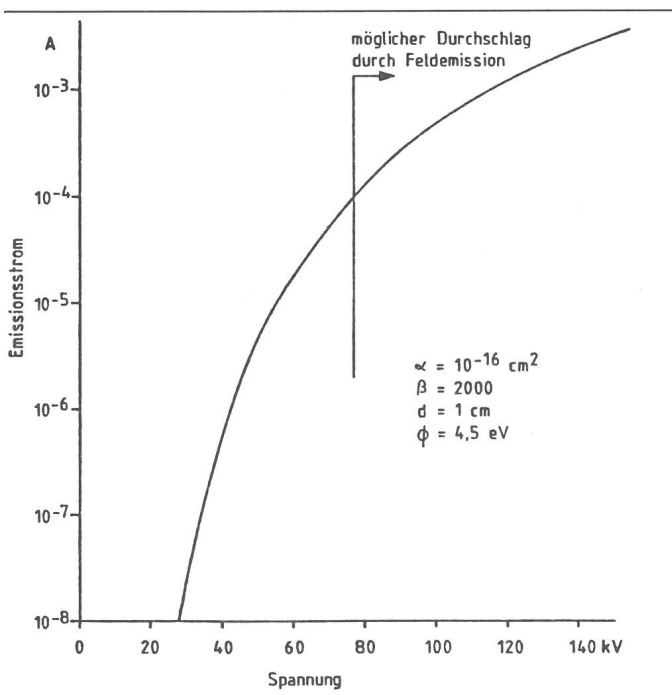
Fig. 1 Stromspannungscharakteristik einer Vakuumisolerierstrecke unter für Vakuumschalter typischen Bedingungen
