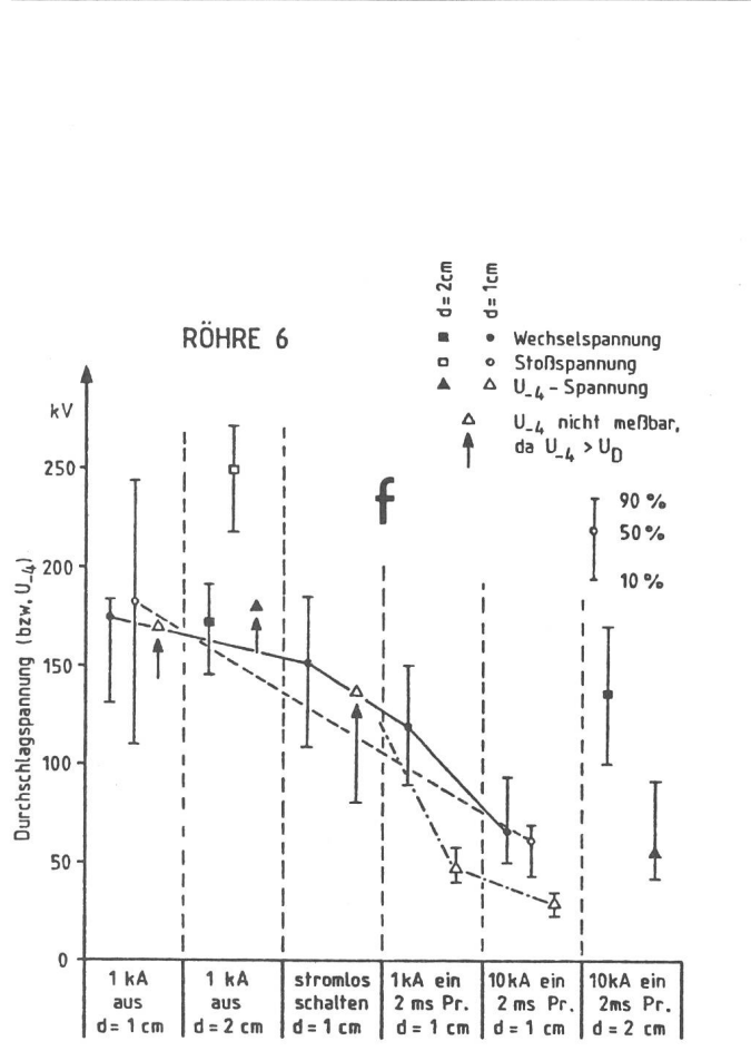
Fig. 2f Wie Fig. 2e, jedoch Kontaktdistanz 10 mm bzw. 20 mm
