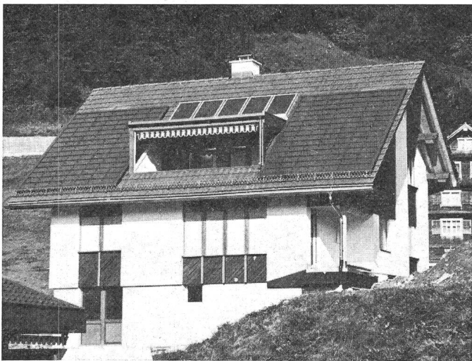
Energiedachanlage mit Absorberflächen und Sonnenkollektoren
