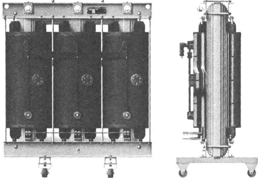
3-Ph-Trocken-Transformatoren RESITRA, lieferbar 50 bis 2'000 kVA, bis 24 kV
