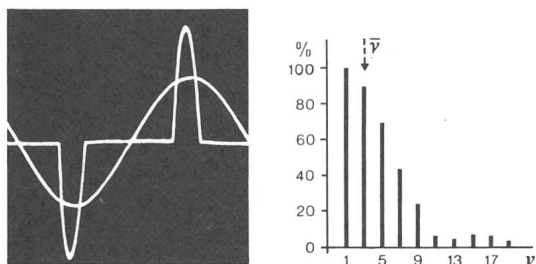
Fig. 8 Belastungsbeispiel Television
