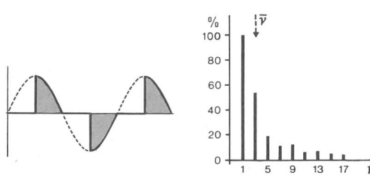
Fig. 11 Belastungsbeispiel Doppelweg-90°-Phasenanschnittsteuerung Ohmsche Belastung
