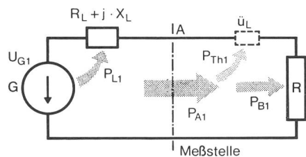
Fig. 3 Grundwellenersatzschema
