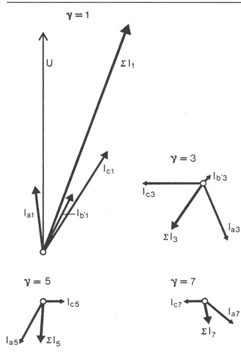
Fig. 12 Vektordiagramm der harmonischen Ströme Belastung (Index) a Television b Fluoreszenzbeleuchtung c 90°-Phasen-Anschnittsteuerung
