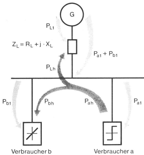
Fig. 5 Verlauf der Leistungsflüsse bei Anwesenheit eines nichtlinearen Verbrauchers a und eines linearen Verbrauchers b im Netz
