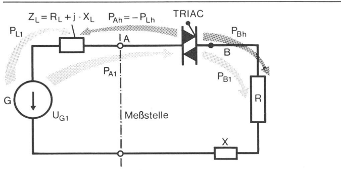
Fig. 2 Verlauf der Leistungsflüsse im Messkreis
