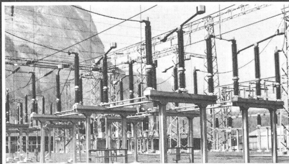
Drehtrenner
