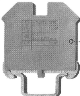
die gleichen Klemmen auch für die 35 mm-Tragschienen nach DIN 46277/3 resp. EN 50022
