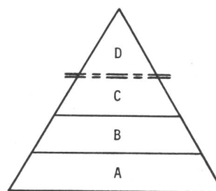
Fig. 4 Niveaux fonctionnels des systèmes d'automatisation à structure hiérarchique A Commande locale C Salle de commande B Automate de groupe D Dispatching régional
