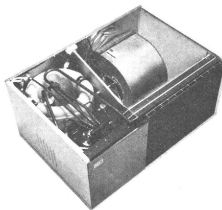
Luft-Wasser-Wärmepumpe LWP 5000
