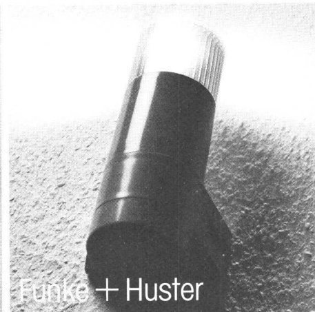
Solarsystem 2000
