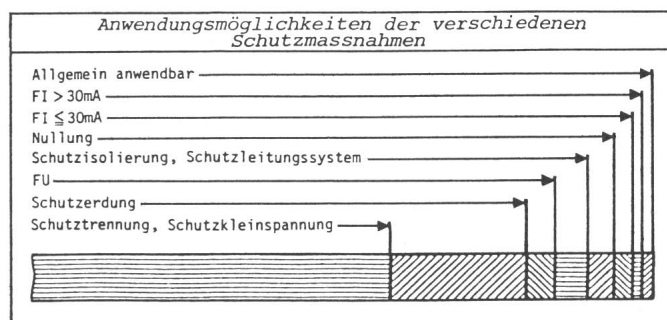
Schutzmassnahmen nach CENELEC-Harmonisierungsdokument 384.4.41
