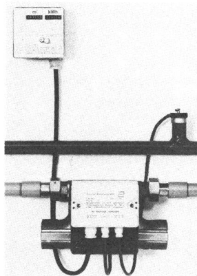
Statischer Wärmehöher WSA mittels Ultraschall (Landis & Gyr)
