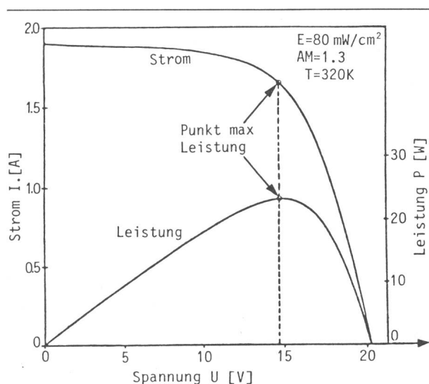
Fig. 2 Gemessene Strom-Spannungs( I-U )- und Leistungs-Spannungs( P-U )-Kennlinie eines Moduls aus monokristallinen Silizium-Solarzellen E ist die Bestrahlungsstärke auf der Modulfläche, AM die Luftmasse (air mass) und T die absolute Temperatur des Modulgehäuses
