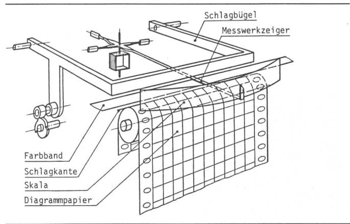
Fig. 8 Prinzip eines Punktschreibers
