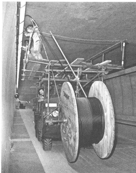
Fig. 5 Abgänderter Lastwagen für die Kabelmontage
