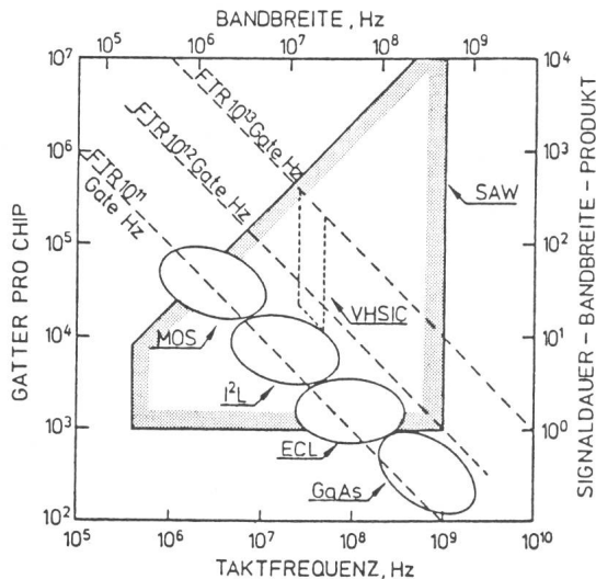
Fig. 1 Vergleich der Signalverarbeitungskapazität von SAW-Komponenten und digitalen integrierten Halbleiterschaltungen
