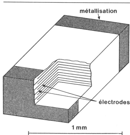
Fig. 9 Condensateur céramique miniature à électrodes métallisées
