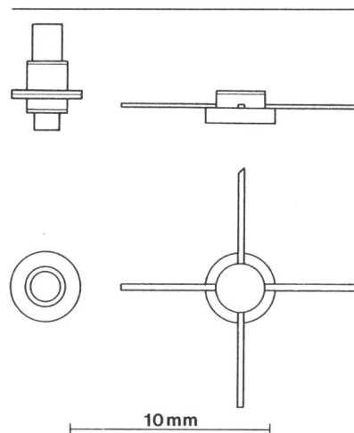
Fig. 11 Transistors pour montage sur circuits microruban
