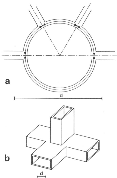
Fig. 2 Jonction hybride a) en lignes microruban; b) en guides d'ondes; la dimension relative est indiquée par d
