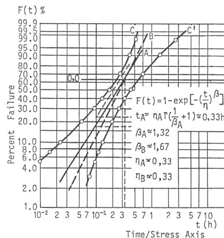
Fig. 5 Résultats des essais à 2,7 U_N
