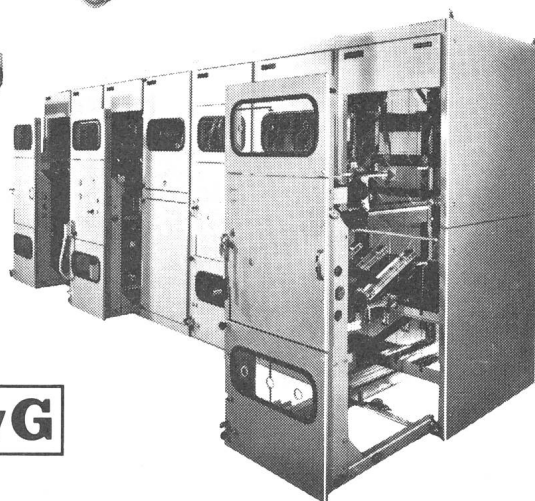
24 kV-Anlage mit Schmalzellen, ölarmer Leistungsschaltern und autopneumatischen Lasttrennern.
