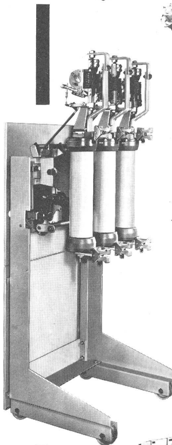
24 kV-Anlage mit Schmalzellen, ölarmer Leistungsschaltern und autopneumatischen Lasttrennern.
