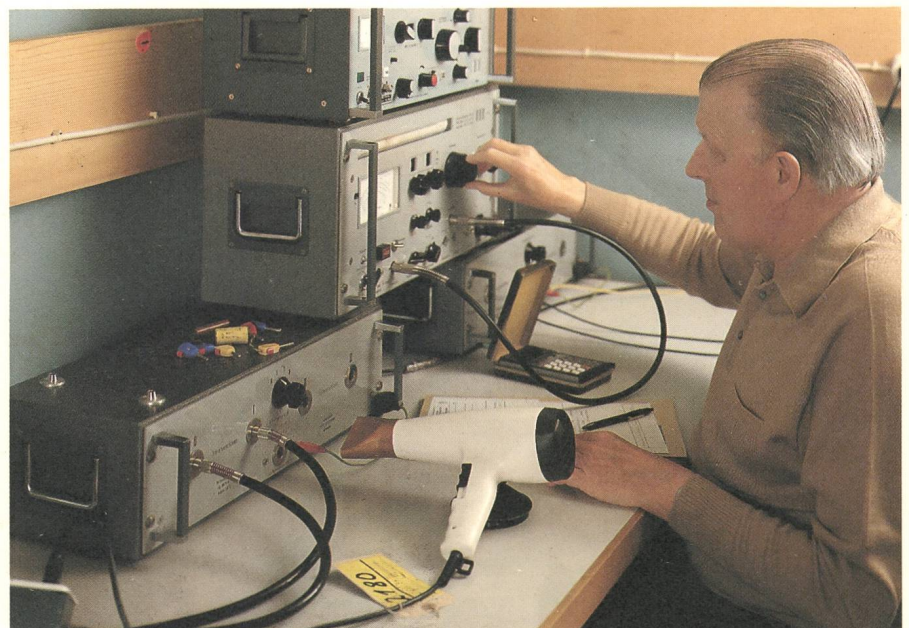
Radiostörschutzmessung an einem Haartrockner
