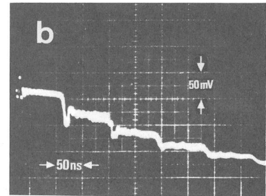
Fig. 4 Ausgangsspannung des NEMP-Generators
