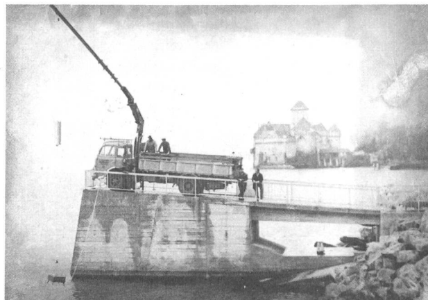
Fig. 6 Mise en place d'un flotteur de l'écran électrique et de son corps-mort
