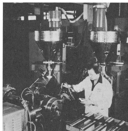
Fig. 10 Co-extrusion von Schichten in Dreifach-Spritzkopf
