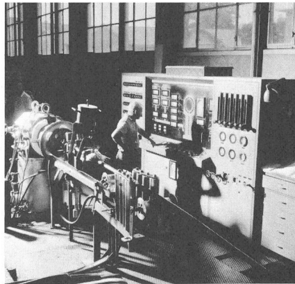
Fig. 16 Hansson-Bleipresse
