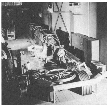
Fig. 6 61spulige Leiterverseilmachine
